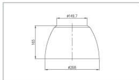
Outdoor Sunvisor (SK-AS01)
